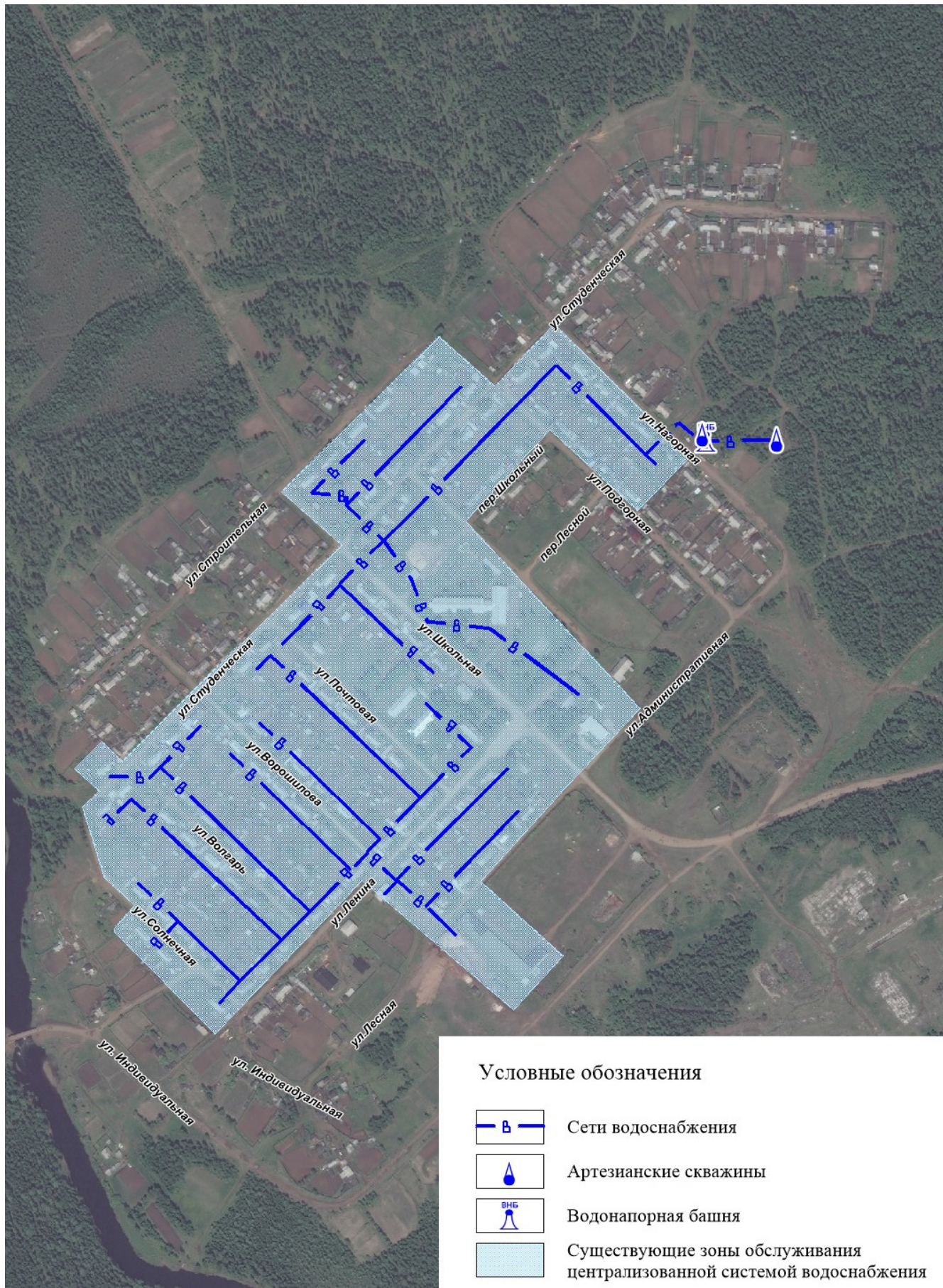
Рисунок 1 - Технологическая зона водоснабжения с указанием зоны обслуживания централизованной системы холодного водоснабжения п. Бадарминск
