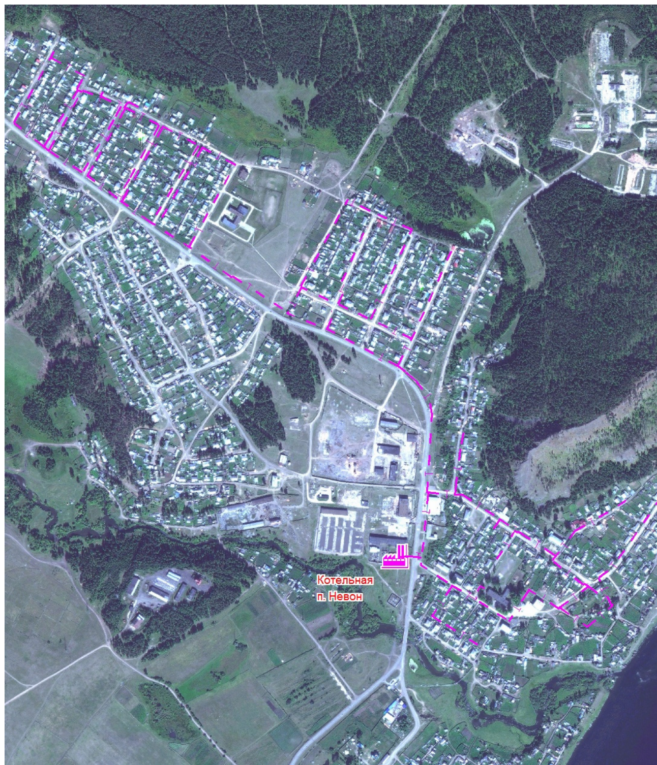
Рисунок 2 – Схема реконструируемых сетей теплоснабжения и реконструируемой котельной п. Невон
