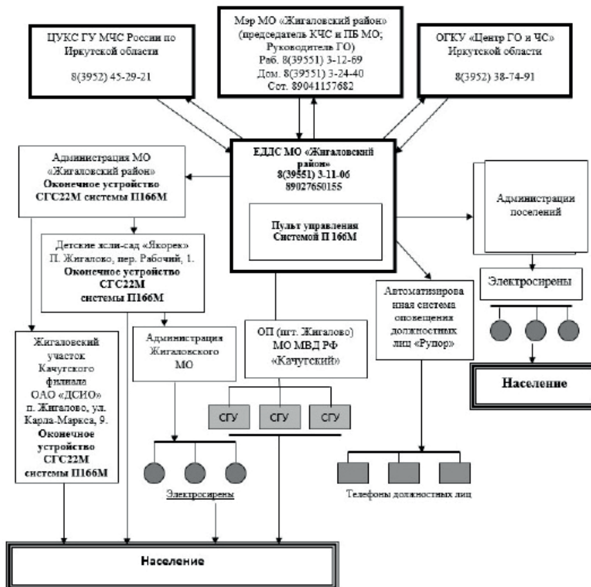
Схема оповещения органов управления, сил гражданской обороны, муниципального звена ТП РСЧС и населения муниципального образования «Жигаловский район»
