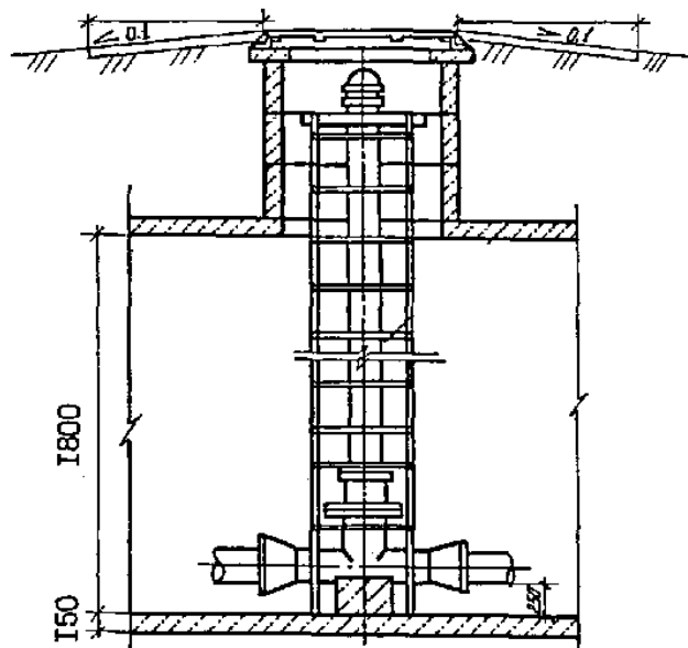
Рисунок 2 – Схема установки пожарного гидранта на водопроводной сети
