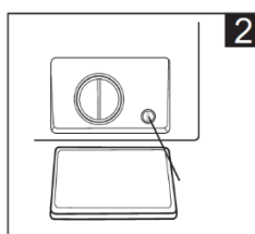
Поверните блокиратор на 90 ° и выгните аварийный сливной шланг.
