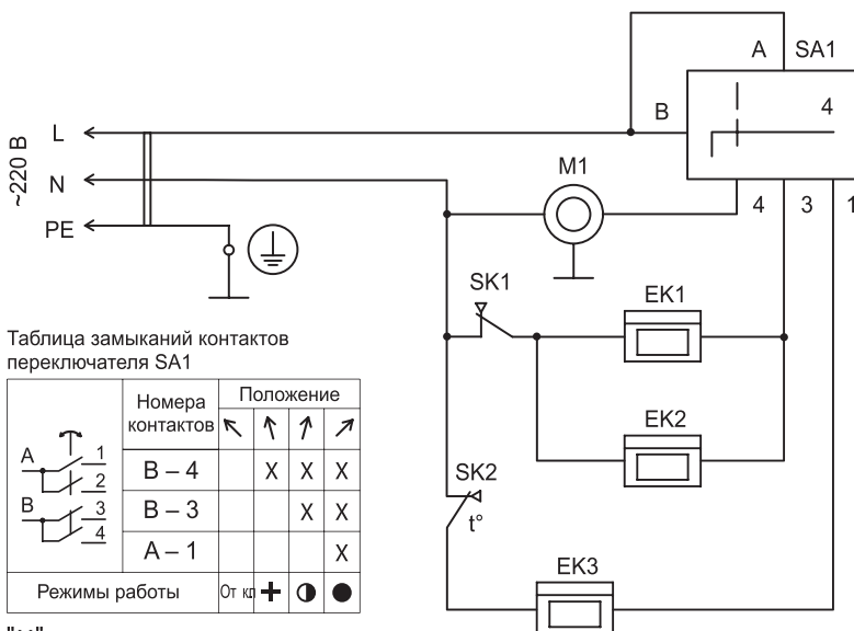
Схема электрическая ТПК-5
