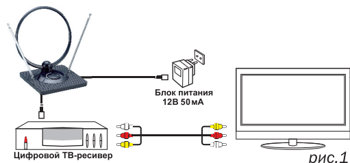
Цифровая антенна
