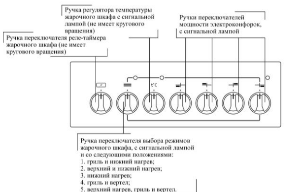
Рис. 13. Передняя панель плиты ЭП43р3
