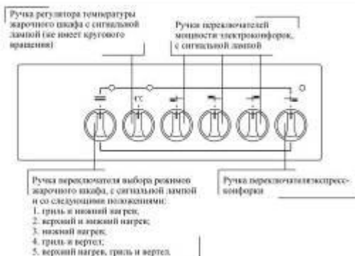
Рис. 11. Передняя панель плиты ЭП41/303
