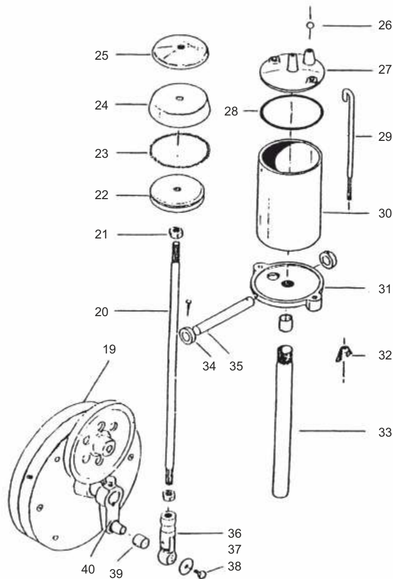
Монтажная схема №3
