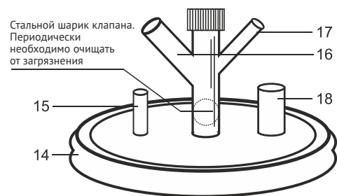
Монтажная схема №2
