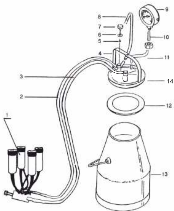
Монтажная схема №1
